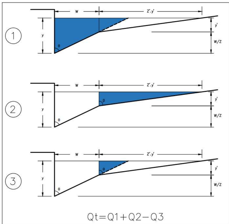
Figura 1 - 3 – Detalhes Hidráulicos da Sarjeta
